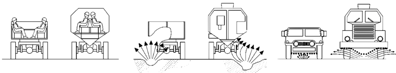
Рисунок 1. Напрямок фугасної дії на автомобілі з прямим і V-подібним днищем
